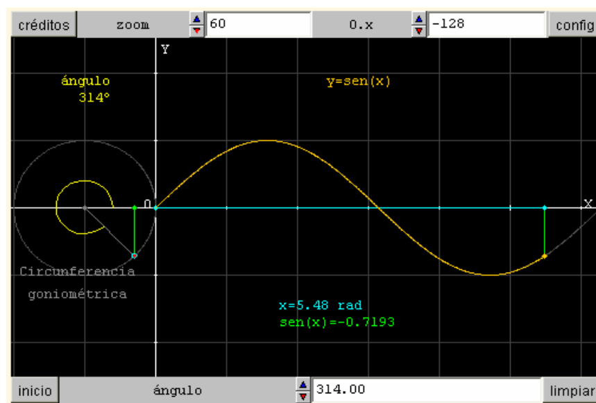
Del círculo trigonométrico a la función trigonométrica en el plano.
