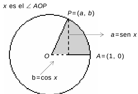
Fig. 2.4 Descripción geométrica de \sin x y \cos x
